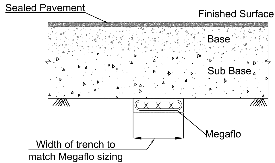
MITRE DRAIN DETAIL (Section A-A)
