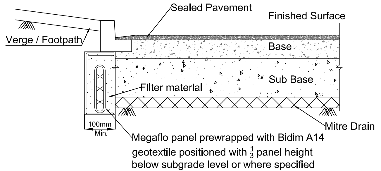
LONGITUDINAL DRAIN DETAIL
